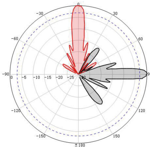
V-Pol
