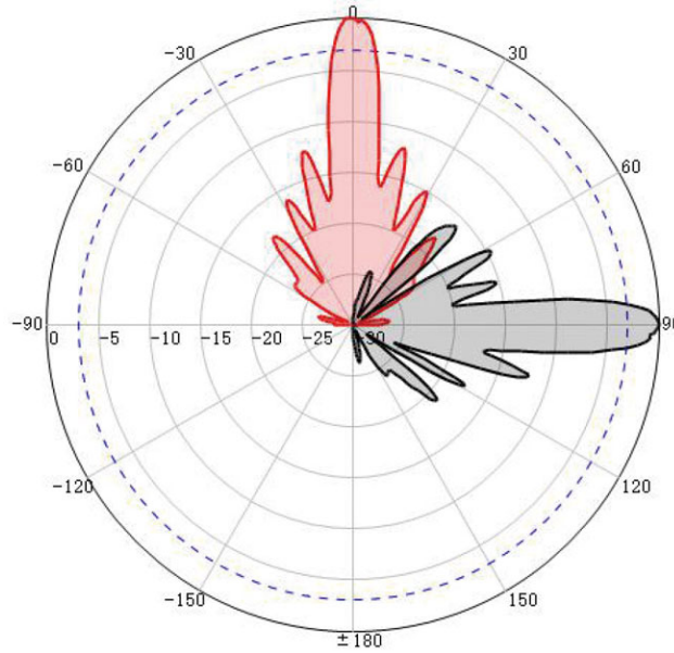
H-Pol
